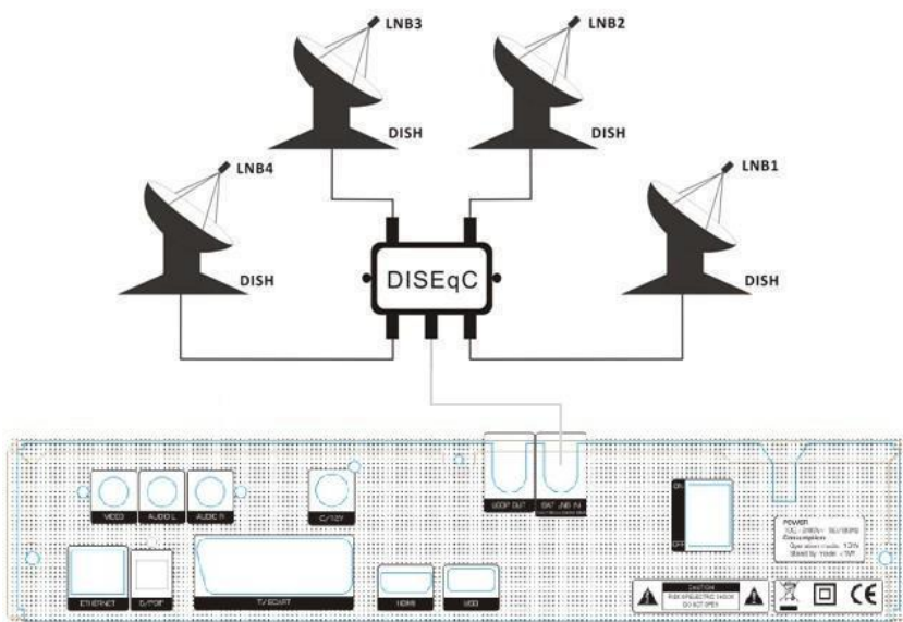
Bild 8. Anschluss an LNB-Satellitenschüssel
