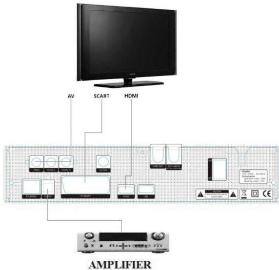
Bild 6. Anschluss an TV & VCR
