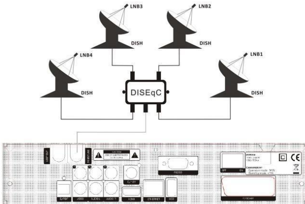
Bild 8. Anschluss an LNB-Satellitenschüssel
