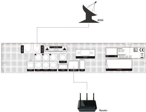
Bild 7. Anschluss an LNB-Satellitenschüssel
