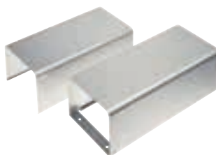
KAMINAUFSATZ FÜR FLACHHAUBEN Kaminaufsatz für Unterbau- Dunstabzugshauben DU 4561, DU 4361, DU 4161, DU 3160 und DU 3150. Ausführung nur in Edelstahl erhältlich.
