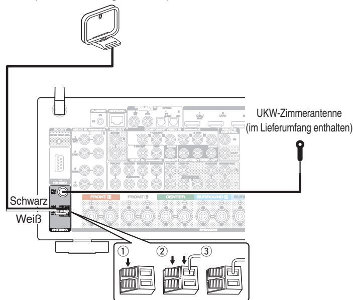
MW-Rahmenantenne (im Lieferumfang enthalten)
