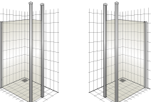
Variante C2L 5, Wandprofil
